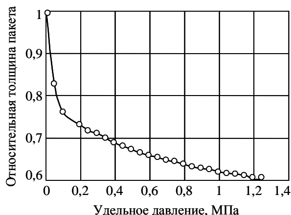
Рис. 1. Изменение толщины пакета ткани в зависимости от величины приложенного давления
