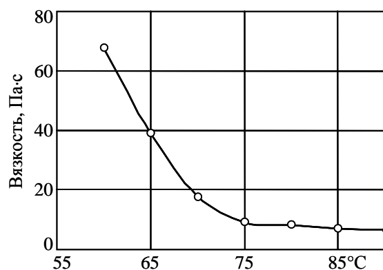
Рис. 2. Температурная зависимость изменения вязкости связующего ВСО-200М
