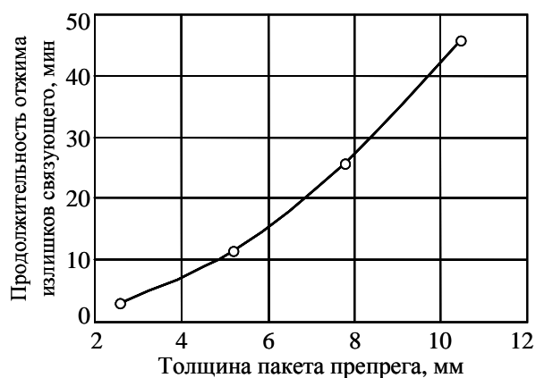
Рис. 4. Изменение продолжительности удаления излишков связующего в зависимости от количества уложенных слоев препрега (расчетные данные)
