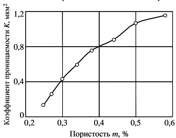
Рис. 3. Зависимость проницаемости стеклоткани от ее пористости
